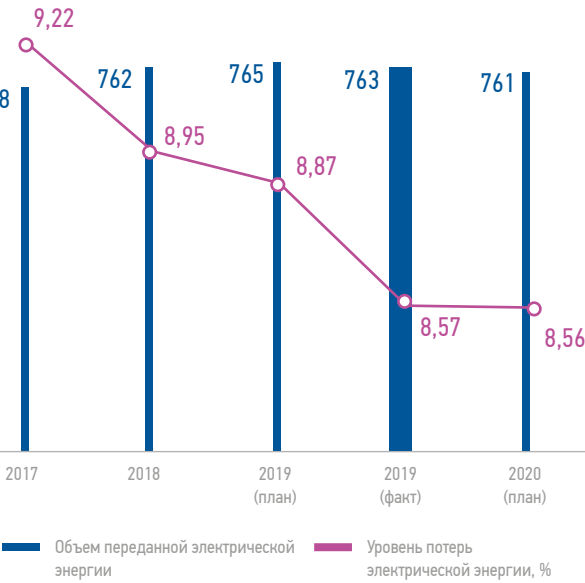
Показатели услуг по передаче электроэнергии, млрд кВт·ч
