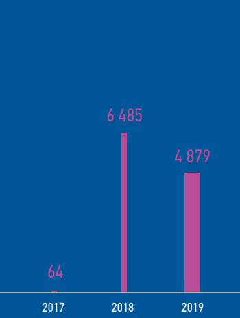
Объем рекультивации нарушенных земель за 2017–2019 гг., га
