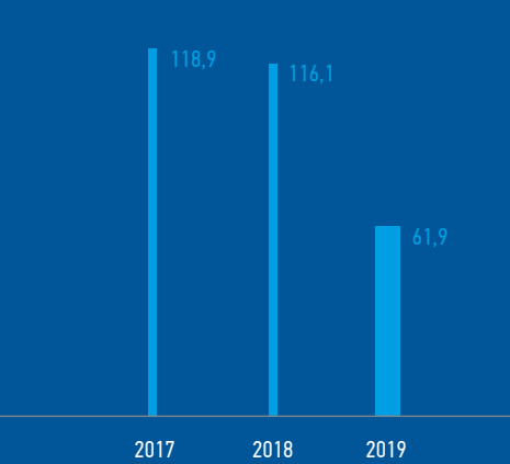
Объем водоотведения в поверхностные водные объекты за 2017–2019 гг., тыс. м³
