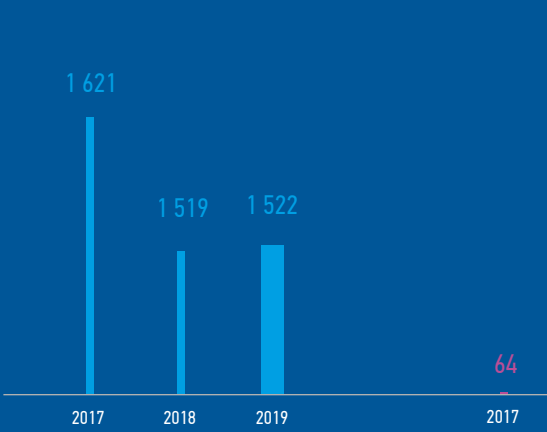
Объем валовых выбросов загрязняющих веществ в атмосферный воздух за 2017–2019 гг., тонн
