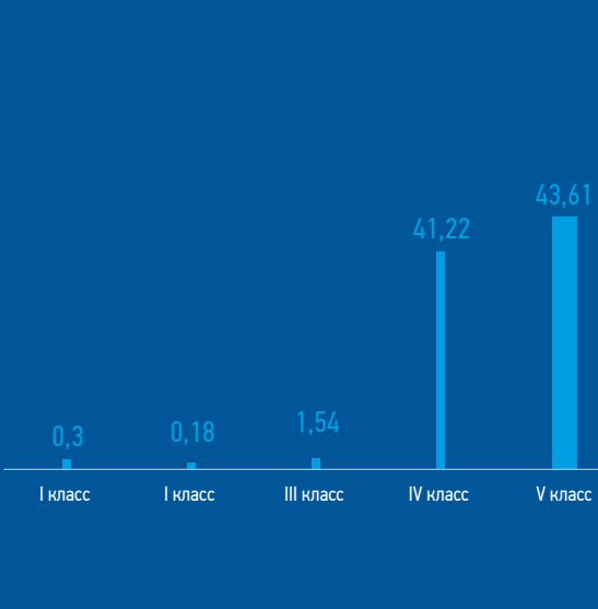
Распределение отходов по классам опасности в 2019 г., тыс. тонн
